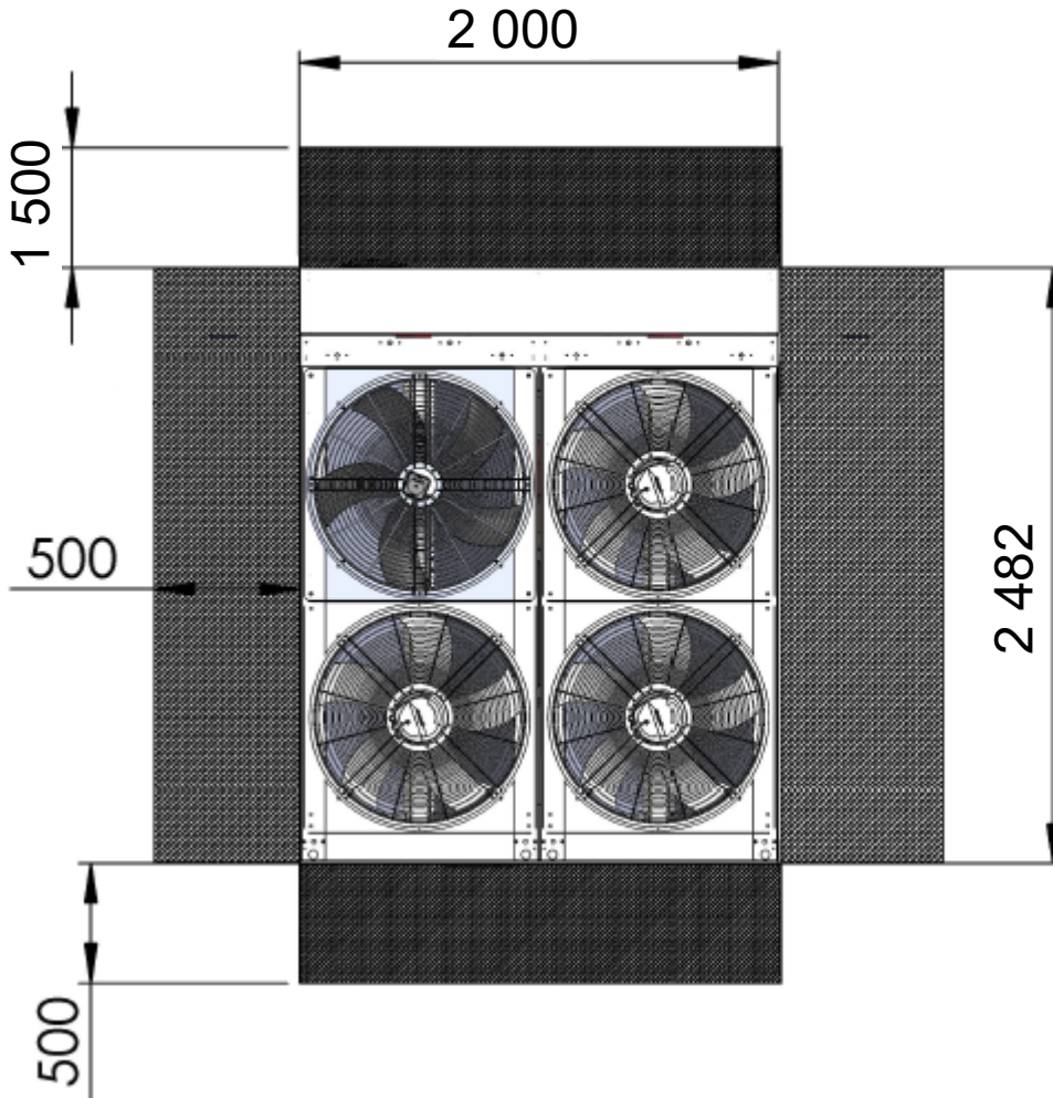
Figure 2 : Dégagements minimum requis [mm]
