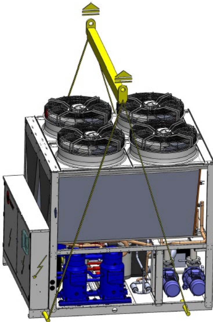
Figure 1 : Procédure de levage
